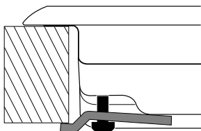
Position der Haken für Arbeitsplatten H=40mm
